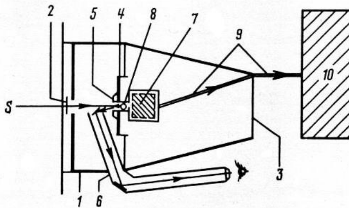
Рис.1. S – наблюдаемое изображение звезды после оптической системы телескопа; 1 - бронзовый кожух спектрометра; 2 – оптическое стекло; 3 – плотный картон; 4 – щель спектрографа, расположенная в фокальной плоскости телескопа перпендикулярно суточному движению, ширина щели 0,2 мм; 5 – зеркальная щечка щели; 6 – визирное устройство; 7 – приемная система: четырехплечный, одинарный, измерительный мост постоянного тока, построенный на сопротивлениях ОМЛТ-5,6 кОм – 0,125 Вт, питающее напряжение 70-80 В; мост помещен в два плотно вставленных один в другой стакана: картонный и алюминиевый; 8 – чувствительный элемент приемной системы, расположенный непосредственно за щелью на расстоянии 5 мм от нее; 9 – провода связи; 10 – блоки питания, корректировки и регистрации. В качестве нулевого индикатора использовался гальванометр М-95, как в работе [2, 3], или самописец Endim 621.01 в режиме работы “потенциометр”.
