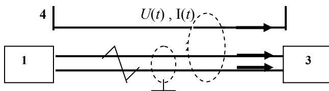
Рис. 5.9. Помехоустойчивая трансляция сигнала по бифилярной линии связи: 1 – источник сигнала; 2 – бифилярная перевитая и экранированная линия связи; 3 – дифференциальный приемник сигнала; 4 – энергетический провод – источник электродинамической и электромагнитной помехи
