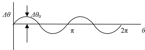
Рис. 3.2. Синусоидальная погрешность СКТ (2-я геометрическая гармоника); \theta – угол поворота вала СКТ; \Delta\theta_0 – предельное значение погрешности.
