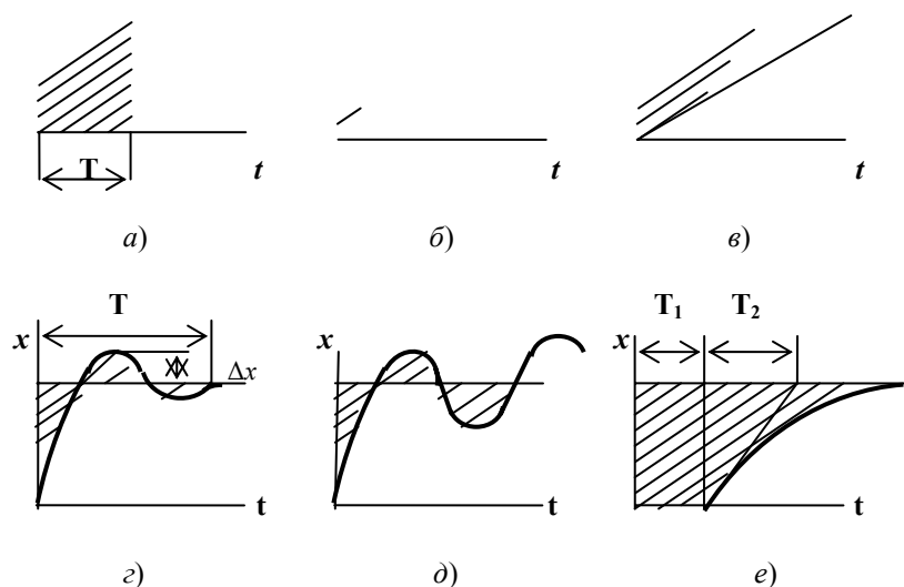
Рис. 2.4. Основные типы переходных процессов при ступенчатом воздействии: а) процесс с запаздыванием; б) экспоненциальный затухающий; в) экспоненциальный расходящийся; г) колебательный затухающий; д) колебательный расходящийся; е) запаздывающий и затухающий; область ошибок заштрихована
