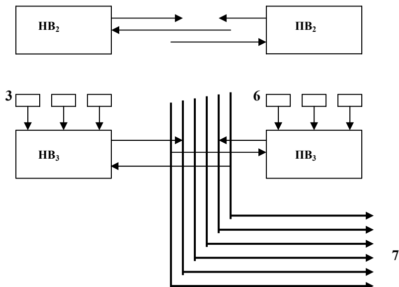
Рис. 5.16. Структура магистрально-радиальной сети связи с ретрансляцией вычислителями первичной информации для пилотажно-навигационного комплекса тяжелого самолета: 1, 2, 3 – комплекты навигационных датчиков; 4, 5, 6 – комплекты пилотажных датчиков; 7 – выход всей пилотажно-навигационной информации к другим потребителям – индикаторам, другим комплексам; NB_1 , NB_2 , NB_3 – комплексные навигационные вычислители; PB_1 , PB_2 , PB_3 – комплексные пилотажные вычислители
