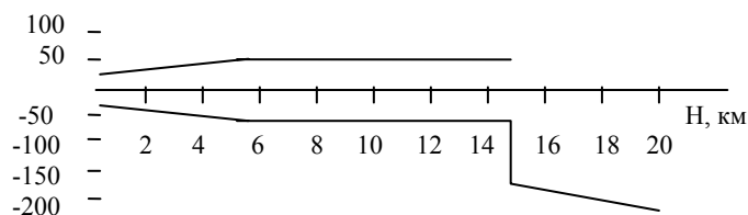
Рис. 2.3. Зависимость значения допустимой погрешности барометрического высотомера от значения высоты.
