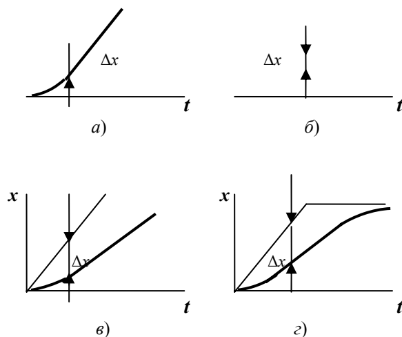
Рис. 2.5. Переходные процессы при изменении целевой функции: а) с постоянной скоростью; б) при изменении целевой функции с постоянным ускорением; в) переходный процесс при наличии звена с ограничением скорости; г) переходный процесс при прекращении нарастания скорости; \Delta x – ошибка системы
