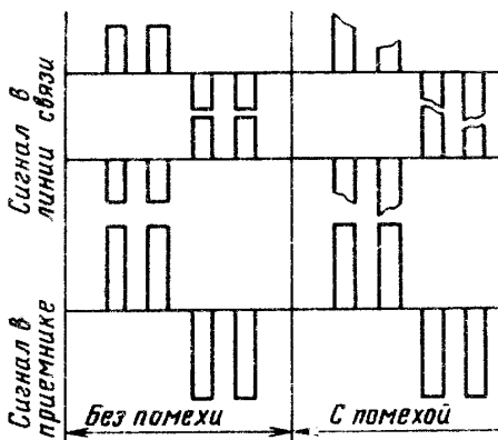
Рис. 1.9. Отделение полезного сигнала от помехи в дифференциальном приемнике сигнала с применением RZ-кода («return tu zero»)
