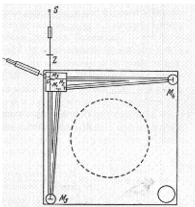
Рис. 3.11. Схема интерферометра Кеннеди
