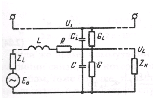
Рис. 1.4. Эквивалентная схема электродинамической связи цепей: U_1 – напряжение в первичной цепи; U_2 – напряжение полезного сигнала; U_n – напряжение помехи во вторичной цепи; C_i, G_i – взаимные удельные распределенные взаимные емкость и проводимость первичной и вторичной цепей; L, R, C, G – удельные распределенные индуктивность, сопротивление, емкость и проводимость вторичной цепи, E_0 – полезный сигнал, z_i – внутреннее сопротивление источника полезного сигнала; z_n – сопротивление нагрузки
