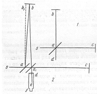
Рис. 1.1. Схема интерферометра А.Майкельсона (Вавилов, с. 28)
