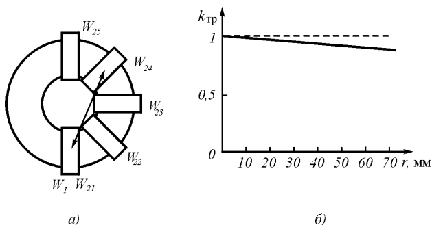
Рис. 3.2. Зависимость относительного значения коэффициента трансформации от взаиморасположения обмоток: a – схема расположения обмоток на кольцевом сердечнике при проведении эксперимента; б – изменение коэффициента трансформации при изменении расстояния между обмотками.
