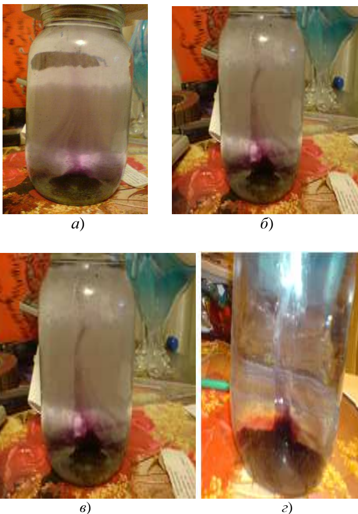
Рис. 2.4. Формирование чернильного вихря в банке с водой после установки на ней деревянного корректора Додоновых: а) через полчаса после установки; б) через час после установки; в) через полтора часа после установки; з) через 15 минут после снятия корректора с банки.
