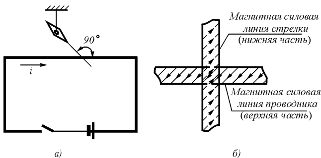
Рис. 4.9. Взаимодействию постоянного тока на магнитную стрелку (опыт Эрстеда): a – схема опыта; б – взаимодействие поля магнитных доменов стрелки и магнитного поля проводника с током
