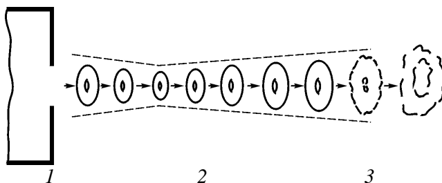
Рис. 6. Формирование газового тороидального вихря с помощью ящика Вуда: 1 – стадия сжатия тороида; 2 – стадия расширения тороида (диффузия); 3 – стадия развала тороида.
