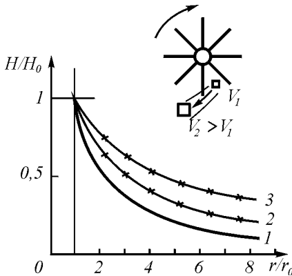
Рис. 2.6. Экспериментальные исследования закона полного тока: a – механическая аналогия – изменение скорости потока сжимаемой жидкости, приводимой в движение вертушкой с лопастями; б – изменение напряженности магнитного поля в зависимости от расстояния от оси проводника; 1 – теоретическая кривая, вычисленная из условия постоянства циркуляции магнитного поля; 2 – экспериментальные результаты при токе I = 1 А; 3 – экспериментальные результаты при токе I = 10 А. Измерения проводились при частотах 50, 400 и 1000 Гц
