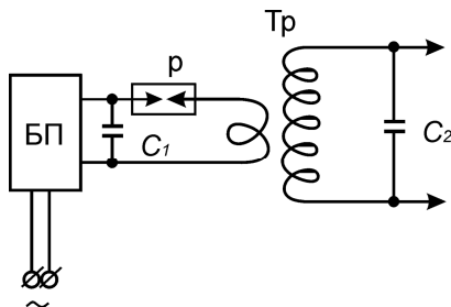
Рис. 16. Схема включения трансформатора Теслы: БП – блок питания; Р – разрядник, C_1 – разрядный конденсатор; Тр – трансформатор Теслы, C_2 – резонансный конденсатор.
