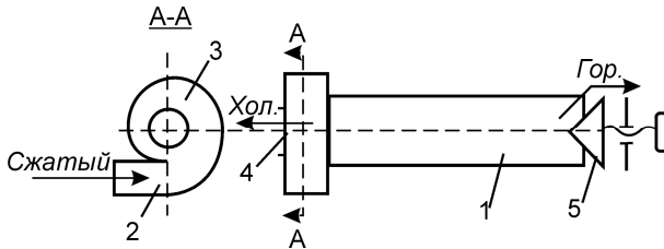
Рис. 6.8. Схема вихревой трубы Ранка
