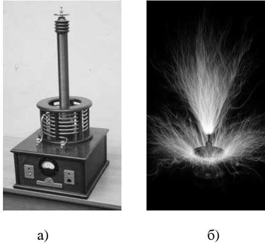
Рис. 17. Трансформатор Теслы: а) общий вид лабораторного образца; б) вид разряда на выходе вторичной (внутренней) обмотки трансформатора
