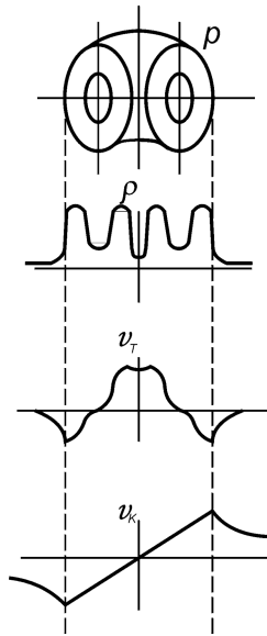
Рис. 10. Структура газового тороидального вихря
