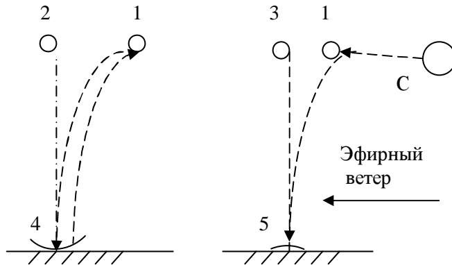
Рис. 1.4. Различные изображения спутника: 1 – истинное положение; 2 – радиолокационное изображение; 3 – оптическое изображение; 4 – радиолокатор; 5 – приемник оптического изображения; С – Солнце.
