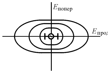
Рис. 5.17. Распространение электрического поля диполем с сосредоточенными параметрами в тонком слое полупроводящей среды. Продольная составляющая больше поперечной составляющей поля
