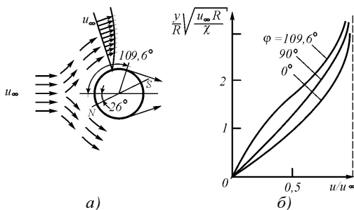
Рис. 1.3. Обтекание шара газовым потоком: а – направление потоков; б – эпоха изменения относительной скорости потока с увеличением расстояния от поверхности шара
