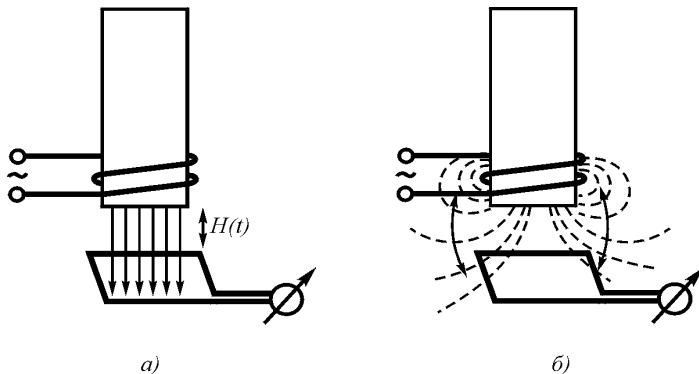
Рис. 5.1. Наведение ЭДС в контуре: а – по Максвеллу; б – в реальности
