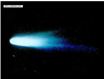
Комета Галлея
