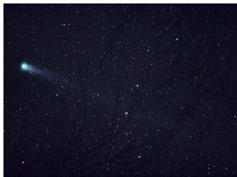
Комета Хиякутаке
