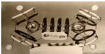
6.2.8. Модель молекулы C_2H_4 электронные пары
