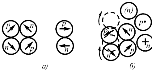
Рис. 6.15. Структура ядра {}^6_3\text{Li}
