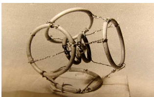
5.2.5. Модель атома углерода
