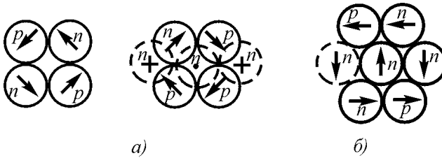
Рис. 1.18. Структура ядер {}^{10}_4\text{Be} (а) и {}^{11}_4\text{Be} (б)
