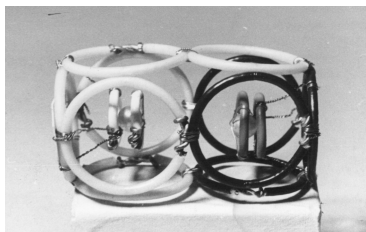
7.2.13. Модель молекулы \text{C}^-\text{O}^+
