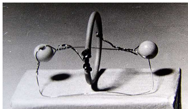
7.2.7. Модель молекулы H 2 +
