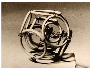
5.2.9. Модель атома аргона
