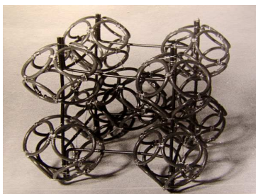
6.3.3. Модель решетки A3
