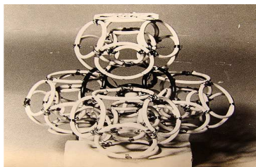
7.4.1. Модель \text{CCl}_4
