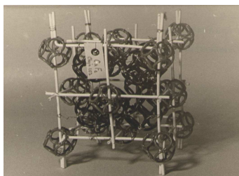
6.5.2. Модель кристалла CaF_2
