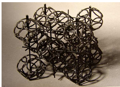
6.3.2. Модель решетки A2
