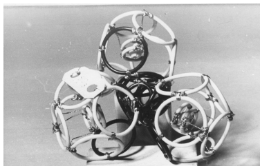
7.2.10. Модель молекулы SO 3
