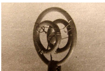
5.2.2. Модель атома лития
