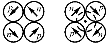
Рис. 1.17. Структура ядра {}^9_4\text{Be}
