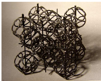
6.3.1. Модель решетки A1
