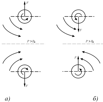
Рис. 1.3. Взаимодействие двух цилиндрических газовых вихрей: a – вращающихся в противоположных направлениях; б – вращающихся в одном направлении
