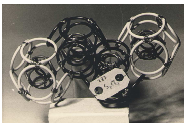
7.4.4. Модель молекулы \text{S}_2\text{Cl}_2
