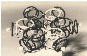
7.3.1. Модель молекулы \text{N}_2\text{H}_4
