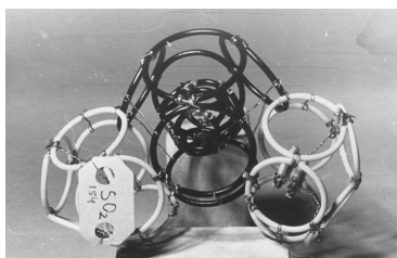
7.2.9. Модель молекулы SO 2
