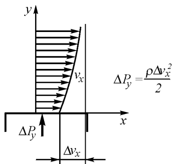
Рис. 4.22. Происхождение поперечной силы, воздействующей на поверхность тела со стороны омывающего потока
