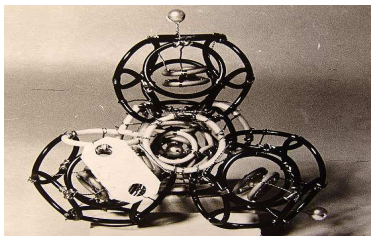
7.2.12. Модель молекулы H 2 SO 4
