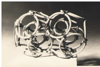
6.2.1. Модель атома Cl 2
