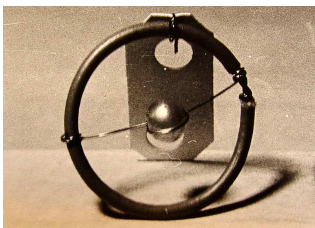
5.2.1. Модель атома водорода
