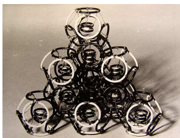
6.4.2. Модель алмаза
