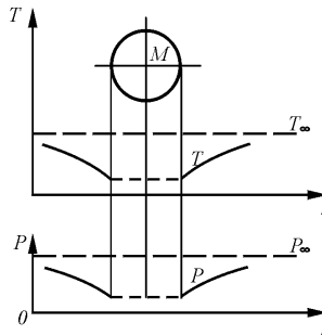
Рис. 4.17. Распределение температуры и давления вокруг совокупности торoidalных вихрей в свободном пространстве
