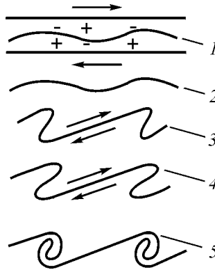
Рис. 4.10. Неустойчивость пограничного слоя между потоками газа: стрелками указаны направления течений; области повышенного давления обозначены знаками +, цифры соответствуют стадиям развития процесса
