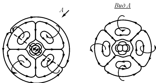
Рис. 2.6. Структура атома лития
