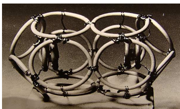
6.2.2. Модель молекулы O 2
