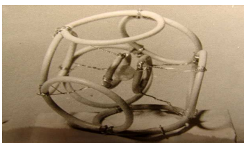
5.2.6. Модель атома хлора
