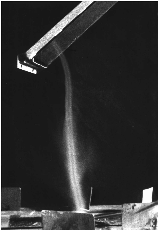
Рис. 4.4. Сжатие газового вихря на входе в воздухозаборник реактивного двигателя самолета (на стоянке)
