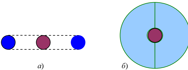
Распределение материи в атоме водорода: а) по Огжевальскому; б) по эфиродинамике.
