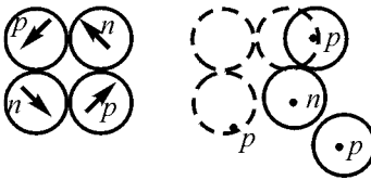
Рис. 1.19. Структура ядра {}_5\text{B}^8
