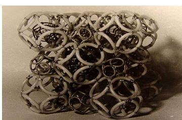
5.2.4. Модель атома бора
