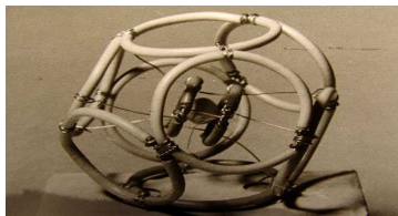
5.2.8. Модель атома неона
