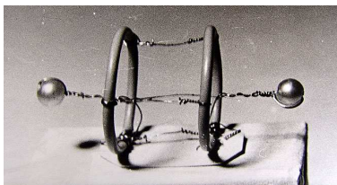
7.2.8. Модель молекулы H 2
