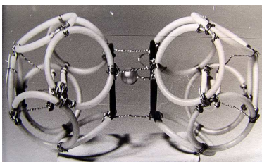
7.2.2. Модель 2\text{H}_2\text{O}
