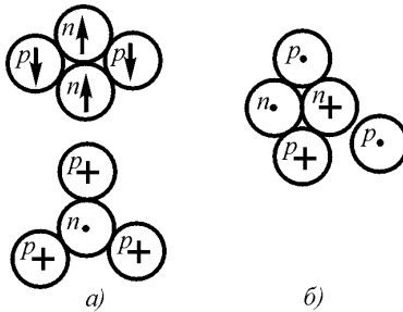
Рис. 1.14. Структура ядра {}^5_3\text{Li} : а – нижний слой; б – верхний слой
