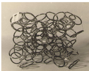
6.4.1. Модель алмаза
