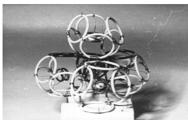
7.2.11. Модель молекулы SO 3 (полимер)
