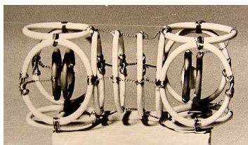
6.2.5. Модель молекулы O 2
