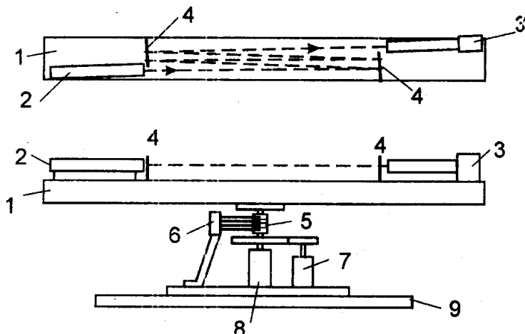
Рис. 9.2. Поворотная лазерная скамья: 1 – жесткая скамья; 2 – гелиево-неоновый лазер; 3 – детектор отклонения лазерного луча; 4 – зеркала с поверхностным отражением; 5 – кольцевой токосъемник для подвода питания и снятия сигнала с детектора; 6 – щетки; 7 – мотор с редуктором; 8 – цилиндрический подшипник скольжения с шаровой опорой; 9 – основание.
