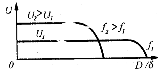
Рис. 7.5. Зависимость сигнала приемника от расстояния между диполями при продольном излучении энергии
