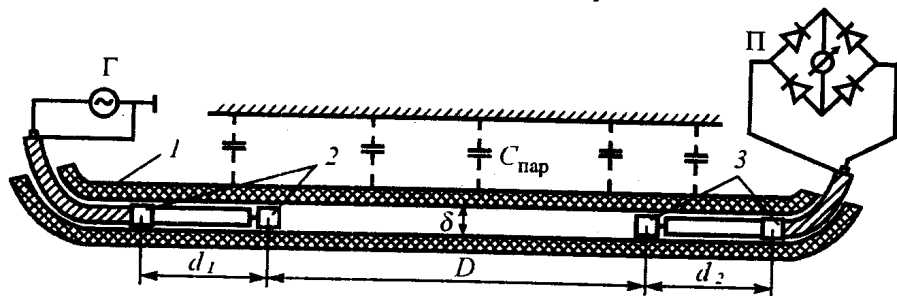
Рис. 7.4. Схема эксперимента по проверке продольного распространения излучения диполя с сосредоточенными параметрами: 1 — резиновый шланг, наполненный подсолонной водой; 2 — электроды излучающего диполя; 3 — электроды приемного диполя; Г — генератор; П — приемник; C_{\text{пар}} — условное обозначение паразитных емкостей
