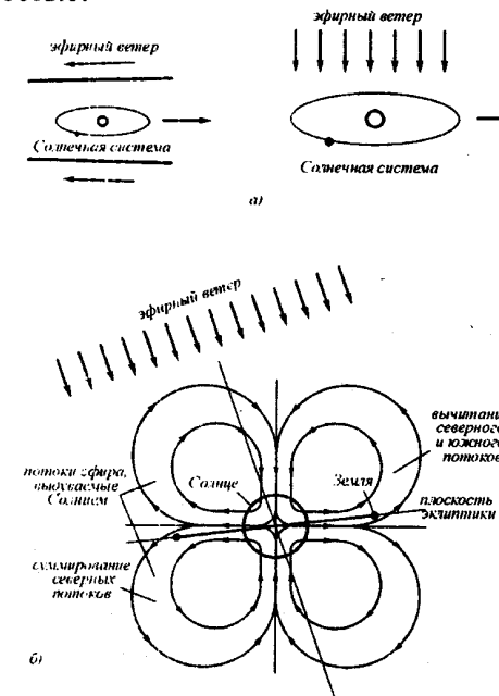
Рис. 12.2. Направление эфирного ветра относительно орбиты Земли: а – в начале образования Солнечной системы и в настоящее время; б – годовые перемещения Земли относительно потоков эфира, создаваемых Солнцем
