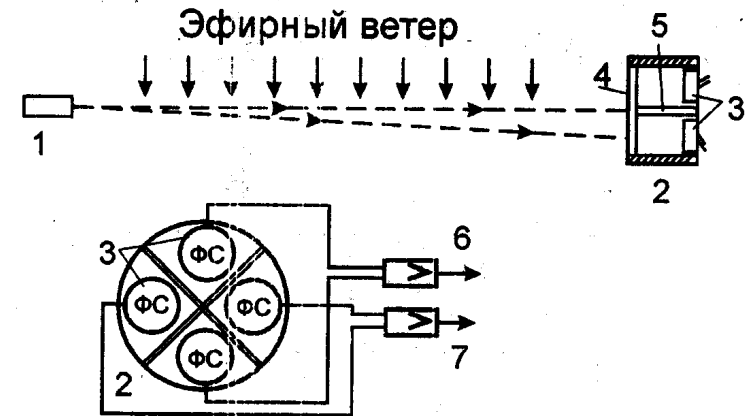
Рис. 9.1. Схема измерения скорости эфирного ветра с помощью лазерного луча: 1 – гелиево-неоновый лазер; 2 – детектор; 3 – фотосопротивления; 4 – матовое стекло; 5 – непрозрачная перегородка; 6 – усилитель сигнала вертикального отклонения луча; 7 – усилитель сигнала горизонтального отклонения луча.
