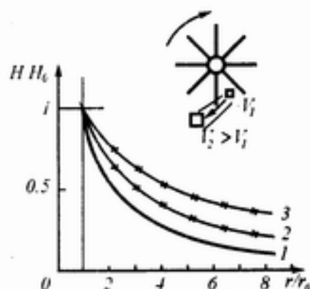
Рис. 2.1. Экспериментальные исследования закона полного тока: a – механическая аналогия – изменение скорости потока сжимаемой жидкости, приводимой в движение вертушкой с лопастями; b – изменение напряженности магнитного поля в зависимости от расстояния от оси проводника; 1 – теоретическая кривая, вычисленная из условия постоянства циркуляции магнитного поля; 2 – экспериментальные результаты при токе I = 1 А; 3 – экспериментальные результаты при токе I = 10 А. Измерения проводились при частотах 50, 400 и 1000 Гц
