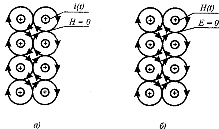
Рис. 5.1. Компенсация полей: а — магнитного поля в распределенной системе токов; б — электрического поля в распределенной системе магнитных потоков
