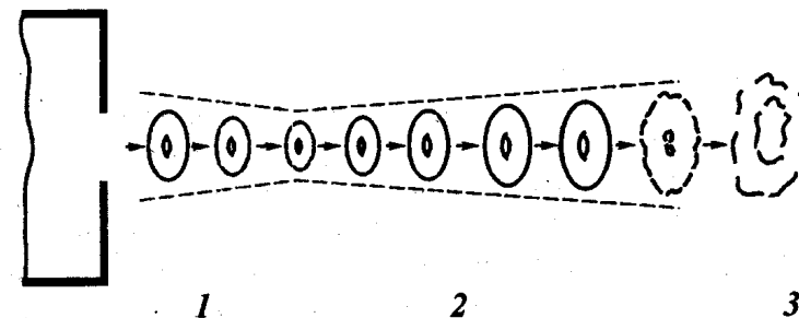
Рис. 8.1. Формирование газового торOIDального вихря с помощью ящика Вуда: 1 – стадия сжатия торOIDа; 2 – стадия расширения торOIDа (диффузия); 3 – стадия развала торOIDа.
