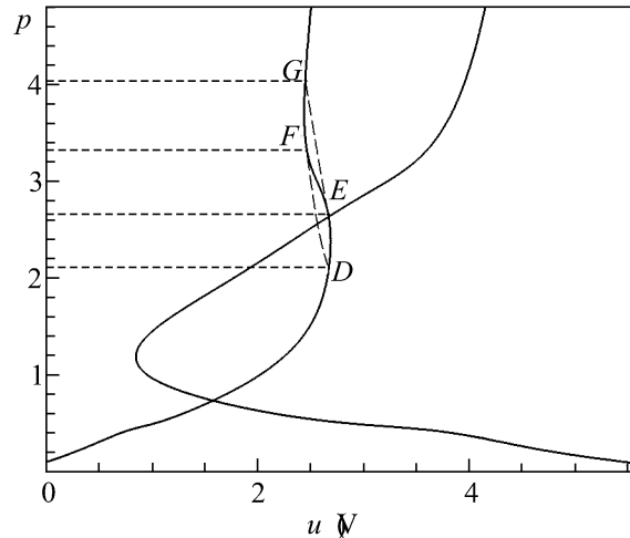
Рис.1. Ударная адиабата с координатами начальной точки p_0 = 0.1 , V_0 = 5.49 , построенная в p-V и p-u координатах на основе УРС (4) при \varepsilon = 10^{-3}
