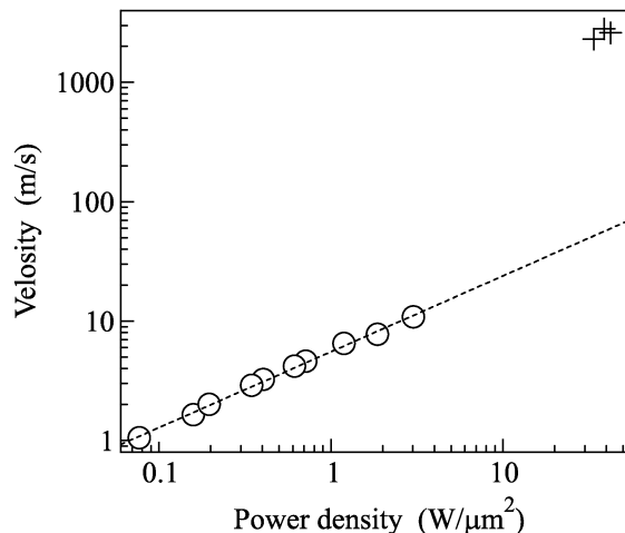
Рис.4. Зависимость скорости движения ОР от интенсивности лазерного излучения. ○ – результаты наших измерений скорости распространения разряда по световоду в режиме медленного горения (в том числе результаты [1]), + – режим быстрого распространения оптического разряда. Пунктир – аппроксимация зависимости V(I) для режима медленного горения ( V = 5.6 \cdot I^{0.635} ), где скорость распространения V в м/с, а интенсивность излучения в \text{Вт}/\mu\text{м}^2 ), экстраполированная в область высоких интенсивностей
