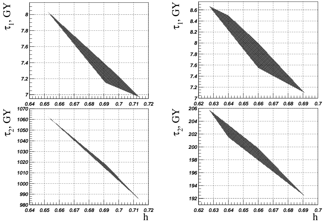
Рис. 2. Возможные значения начала ( \tau_1 ) и конца ( \tau_2 ) ускоренного расширения Вселенной от величины постоянной Хаббла h ; \Omega_{tot} = 1,04 ; 13,5 < \tau_0 < 13,9 GY; 0,126 < \omega_m < 0,143 при \nu = 0,05 (графики слева) и \nu = 0,2 (графики справа).
