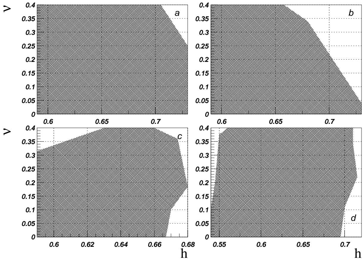
Рис. 4. Области возможных значений постоянной Хаббла h и параметра квинтэссенции \nu при наложении различных экспериментальных ограничений (см. в тексте).
