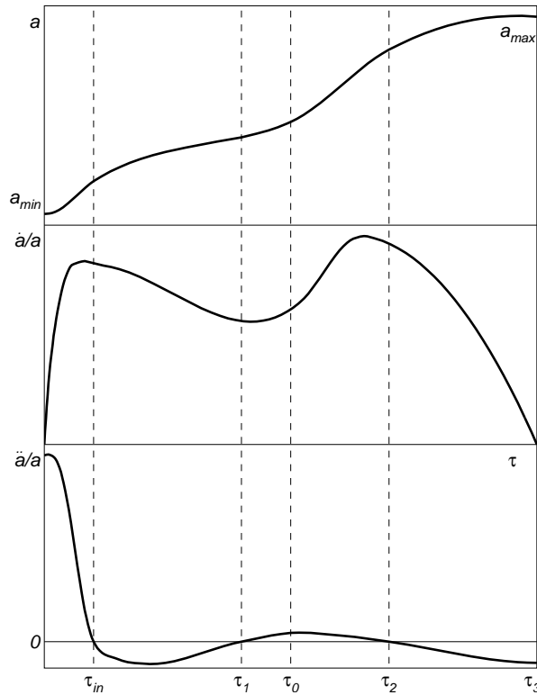
Рис. 1. Качественные кривые зависимости масштабного фактора (вверху), скорости и ускорения (внизу) в зависимости от времени \tau . Здесь \tau_{in} = 1,15\tau_r . Через \tau_0 обозначен современный момент времени. Вначале масштабный фактор от своего минимального значения a_{min} увеличивается с очень большим ускорением, которое за достаточно короткое время \tau_{in} обращается в ноль. Скорость в этот промежуток времени увеличивается от нулевого значения до максимального. Масштабный фактор в течение этого промежутка времени изменяется незначительно: a(\tau_{in}) = \sqrt{2}a_{min} . Далее происходит расширение с отрицательным ускорением, которое обращается в некоторый момент времени \tau_1 в ноль. Значение скорости при этом падает и несколько позже \tau_1 она достигает своего минимального значения. Масштабный фактор на этом отрезке времени продолжает возрастать (расширение продолжается). Движение с положительным ускорением продолжается до момента времени \tau_2 . Скорость и масштабный фактор при этом увеличиваются. При \tau > \tau_2 опять происходит расширение с отрицательным ускорением до тех пор, пока в момент времени \tau_3 расширение останавливается. Масштабный фактор достигает при этом своего максимального значения. На этом полуцикл завершается и все повторяется в обратном порядке — эпоха расширения сменяется эпохой сжатия. Для величины \dot{a}/a первый максимум расположен при a = \sqrt{3/2} a_{min} ( \tau \sim 0,76 \tau_r ) несколько ранее \tau_{in} , точно так же, как второй максимум — ранее \tau_2 . Минимум \dot{a}/a , наоборот, располагается позже \tau_1 . Это следует из того, что величина \frac{d}{d\tau} \left( \frac{\dot{a}}{a} \right) = \frac{\ddot{a}}{a} - \frac{\dot{a}^2}{a^2} при \ddot{a} = 0 отрицательна.
