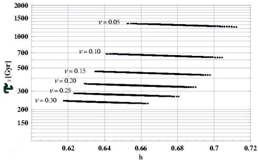
Рис. 3. Зависимость времени максимального расширения Вселенной от величины постоянной Хаббла h для различных значений \nu при \Omega_{tot} = 1,04 ; 13,5 < t_0 < 13,9 GY; 0,126 < \omega_m < 0,143 .
