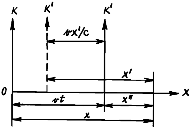
Рис. 1. Координатные системы
