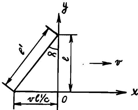
Рис. 3. Искажение углов
