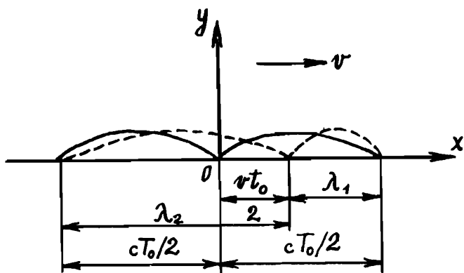
Рис. 5. Эффект Доплера
