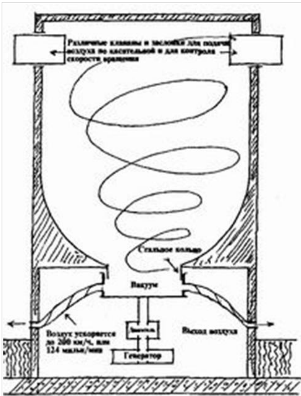
Рис. 21. Импульсионная машина, работающая на воздухе
