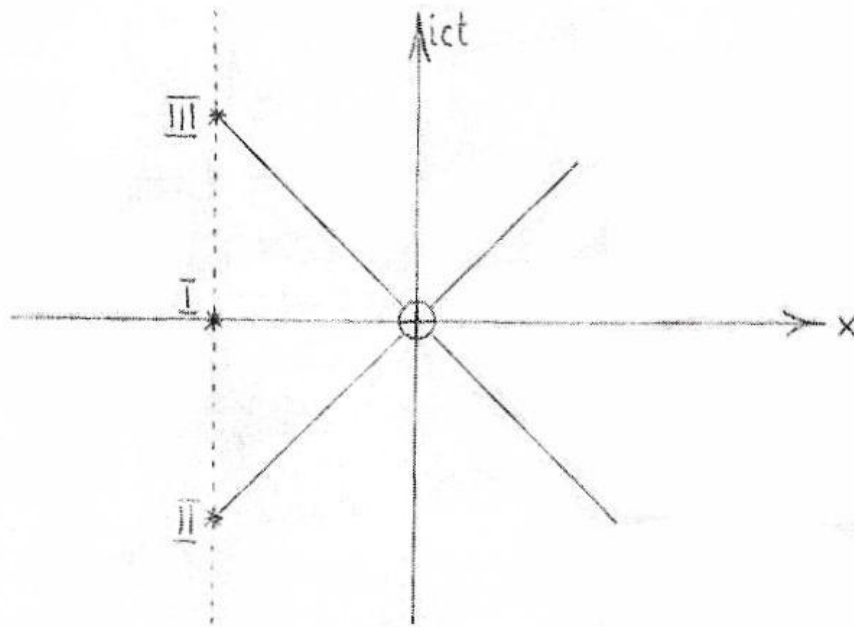
Рис. 1. Три случая возможной связи через время в Мире Минковского.
